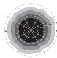
Ansbereich Deckenmontage (Einheit: m) Empfohlene Montagehöhe: 2.5 - 6m
