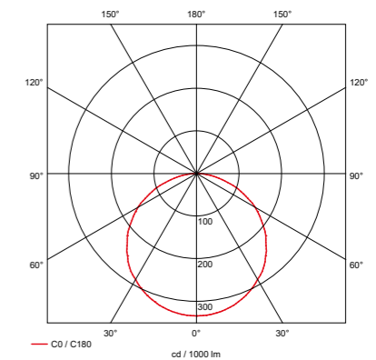
I-Panel Vierkant
