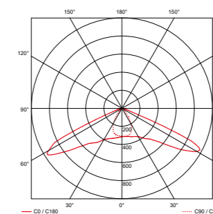
60°x135° asymmetrisch lens
