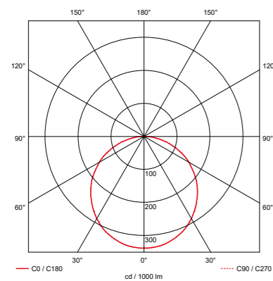
I-Panel Rechthoekig
